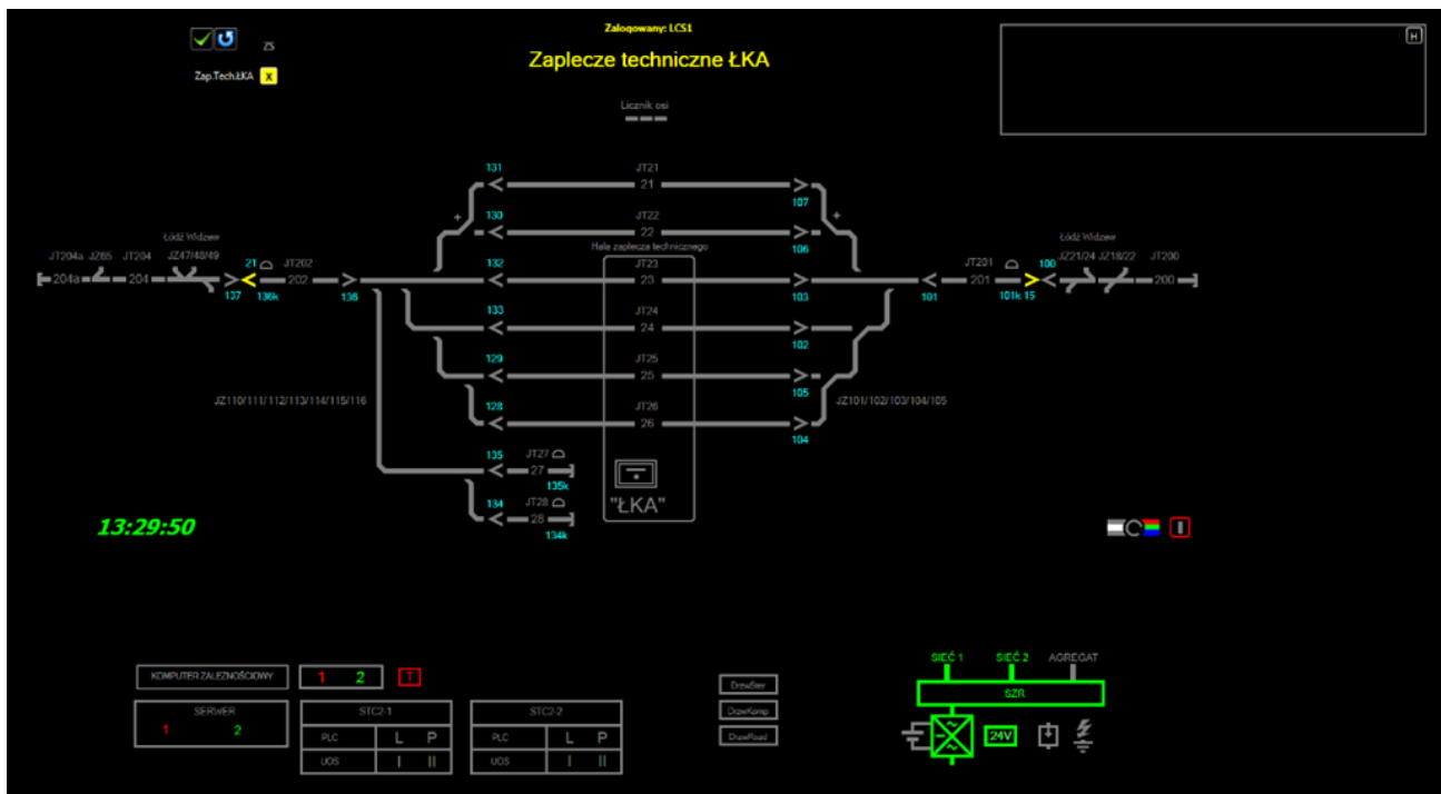
Rys. 15. Obraz stacji (bocznicy) na monitorze systemu EBI Screen 300
