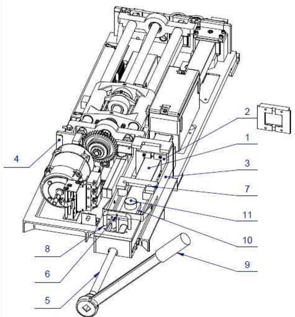
Rys. 46. Pomiar siły rozprucia
