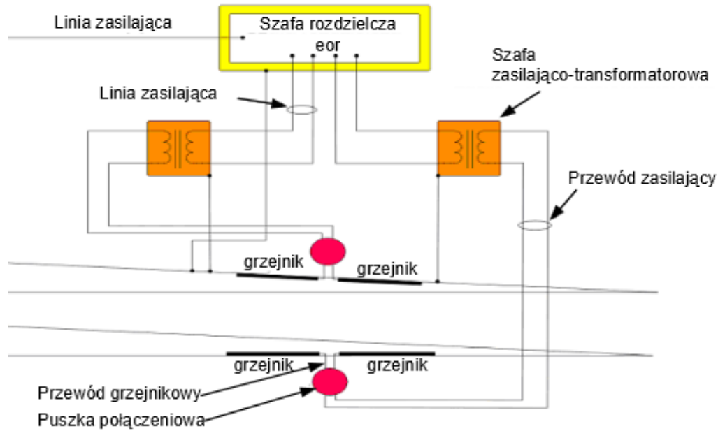
Rys. 47. Schemat ideowy urządzeń eor
