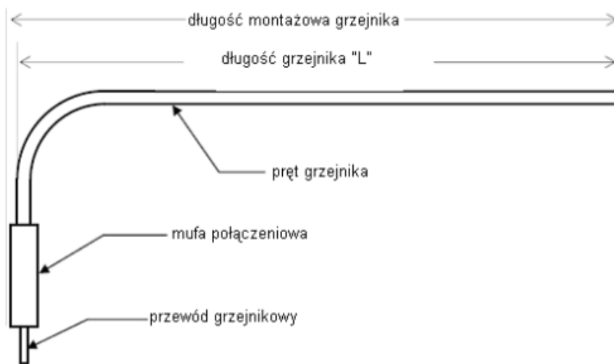
Rys. 49. Schemat grzejnika opornicowego.
