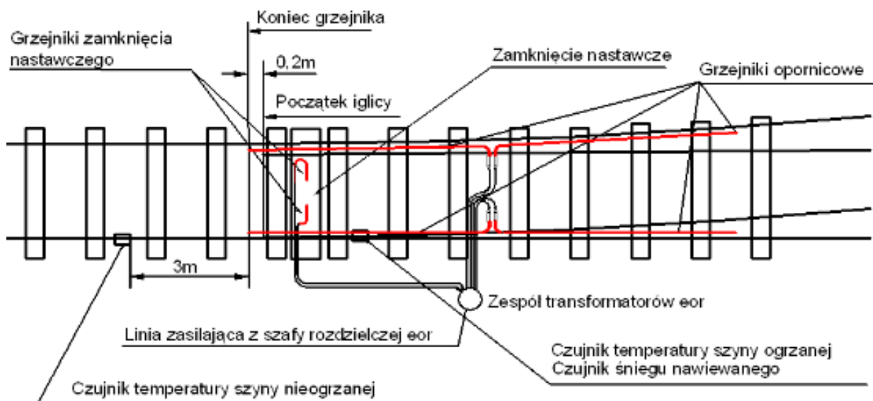
Rys. 48. Instalacja urządzeń eor w rozjeździe
