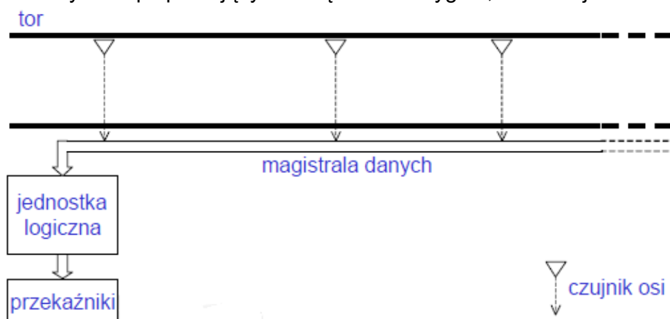
Rys. 5. Schemat blokowy systemu licznika osi
