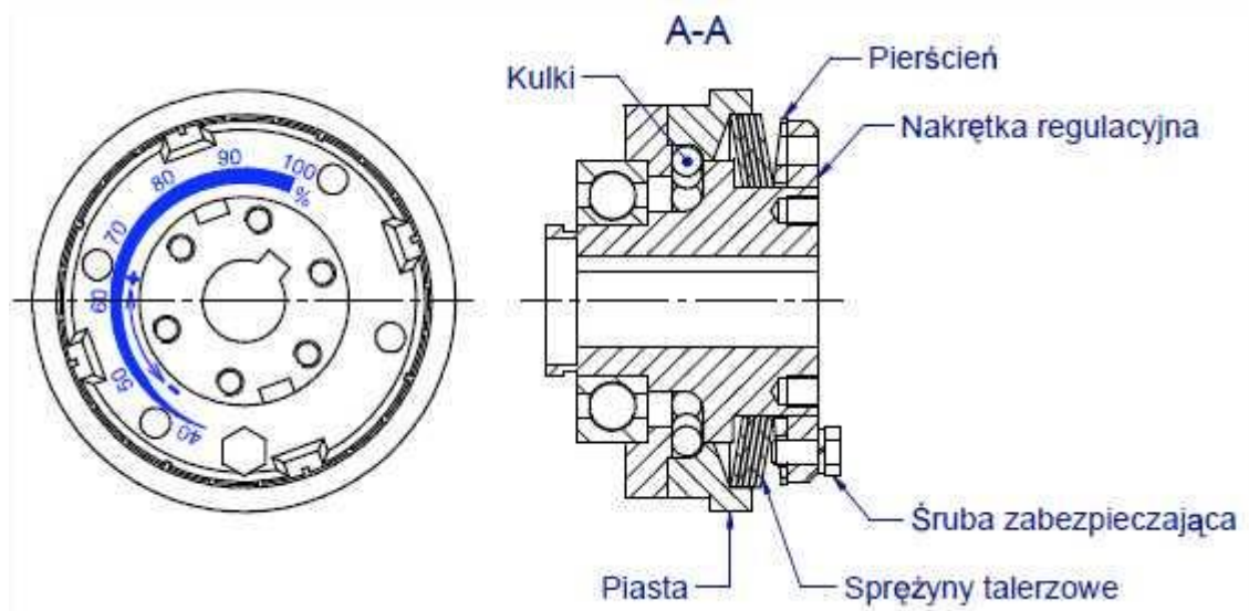
Rys. 45. Sprzęgło EAS-comp.01/490.720.0
